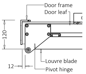
PIVOT JAMB
