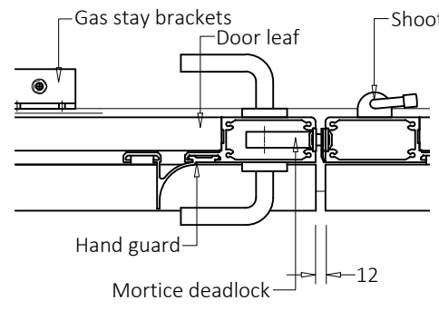
DOUBLE DOOR LOCK
